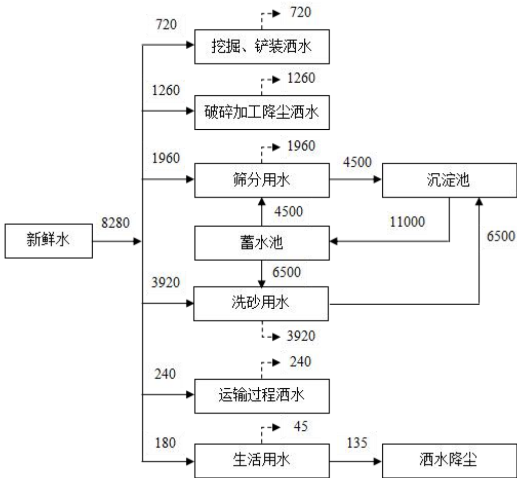
图 3-3 本项目工程用、排水平衡图 (单位: m³/a)
