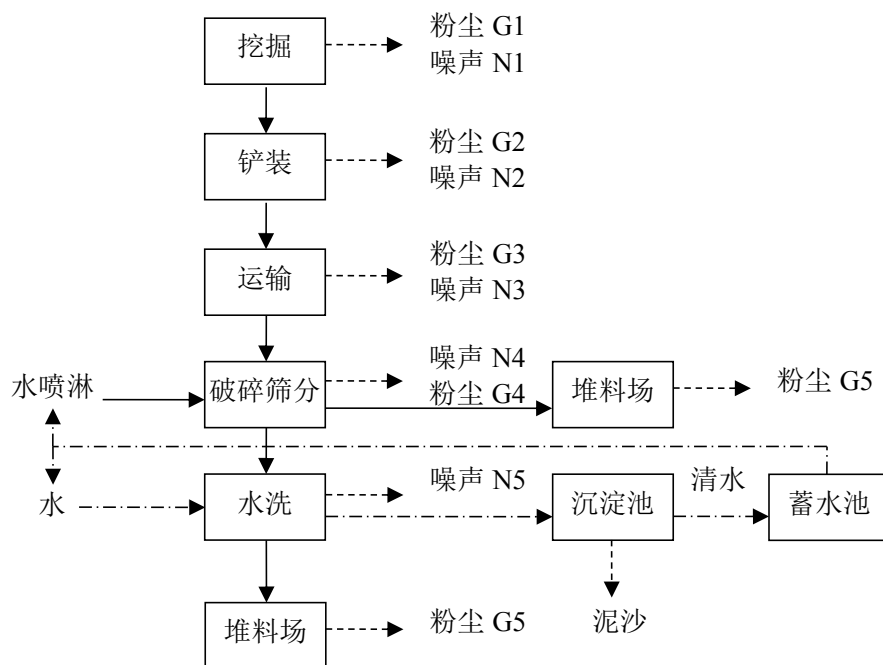
图 3-4 环评阶段生产工艺及产污环节图
